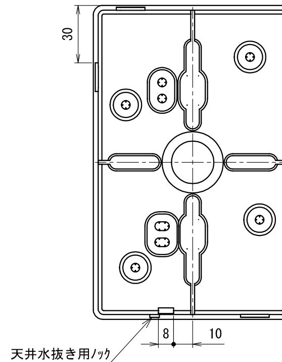
断面 A-A
